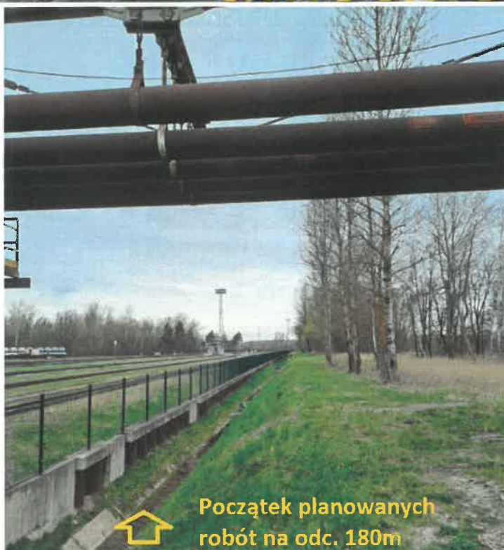
Rys. 1 Rów opaskowy na wysokość rurociągu odpopielania.
